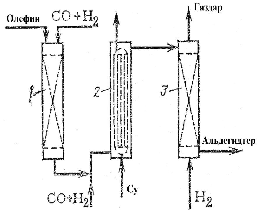
Оксосинтездің үшреакторлы блогы 1, 2, 3 – колонналық реакторлар
