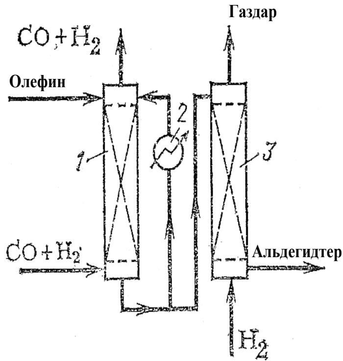
Оксосинтездің екіреакторлы блогы 1, 3 – колонналық реакторлар; 2 – суытқыш
